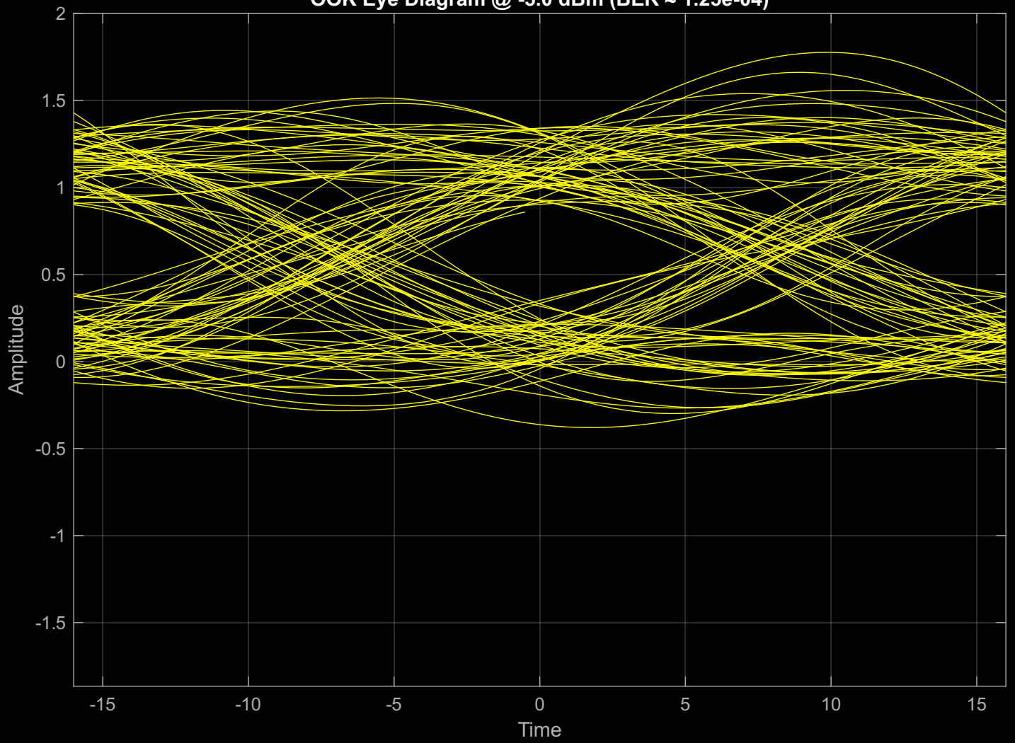
OOK Eye Diagram @ -5.0 dBm (BER \approx 1.25\text{e-}04 )
